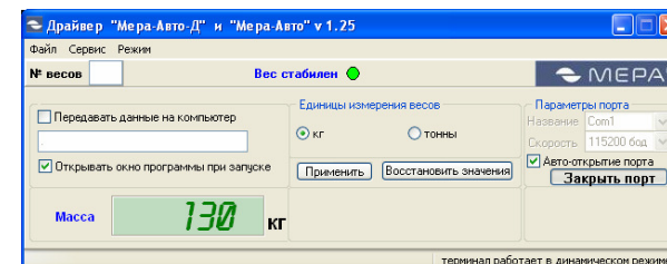
Рис. 5 Рабочая панель в режиме статического взвешивания
