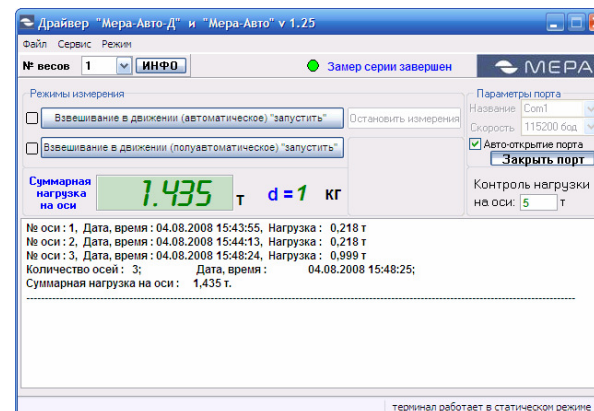
Рисунок 8 – Вид панели в режиме определения суммарной нагрузки на дорожное полотно от всех осей автомобиля.
