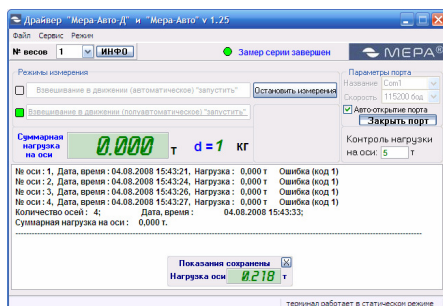
Рис. 7 Индикация нагрузки на одиночную ось или группу осей
