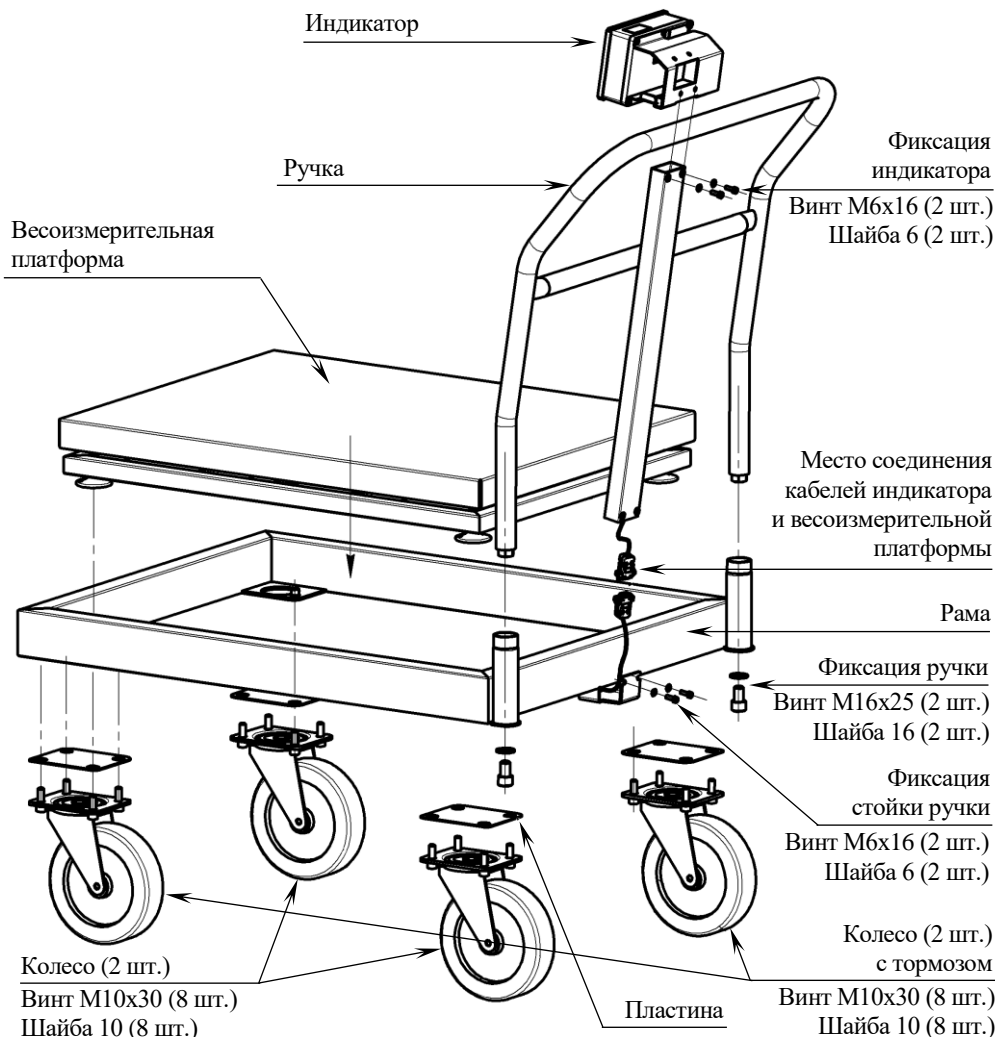
Рисунок 1 – Схема сборки (вид сзади)
